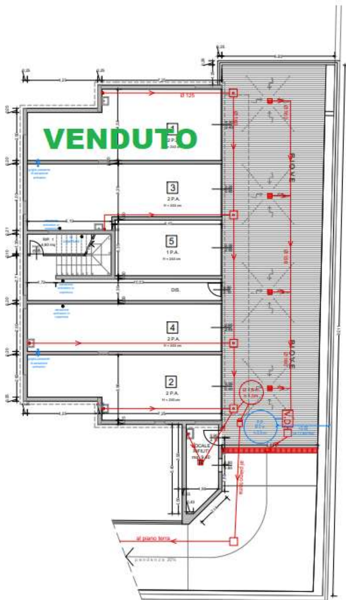
PIANTA PIANO INTERRATO - scala 1:100
